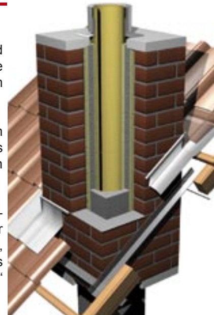
Schornsteinkopf, ummauert
