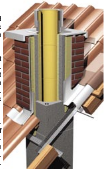
Schreyer Schornstein-Fertigkopf
