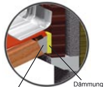
Beton Detail Dachdurchführung mit Betonkranz
