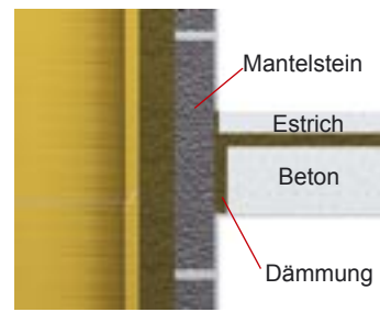
Detail Deckendurchgang
