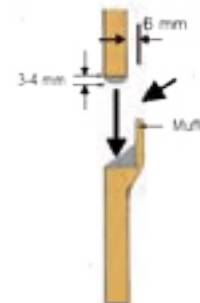
Detail Deckendurchgang
