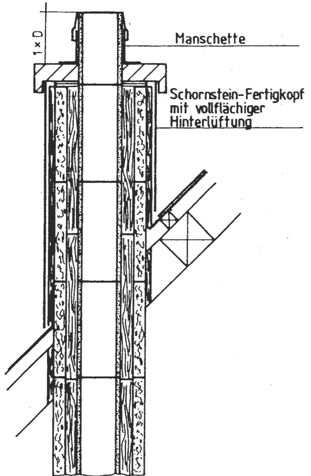
Alternativ - Schornsteinkopf
