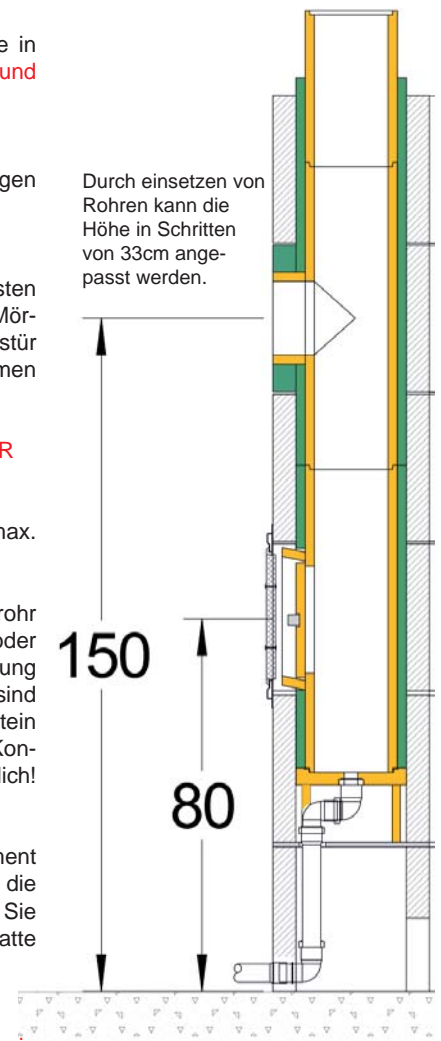
Schreyer FUMDS mit Konsolzylinder
