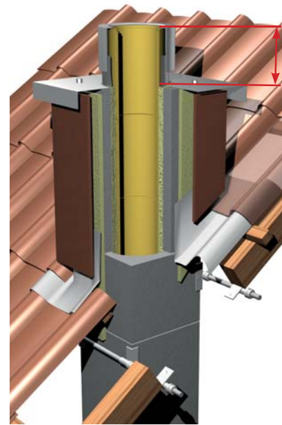
Schreyer Schornstein-Fertigkopf mit Sparrenhalter
