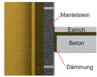
Detail Deckendurchgang
